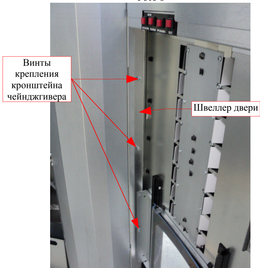
Фото 8а (вид с обратной стороны при закрытой двери защитного кожуха)
